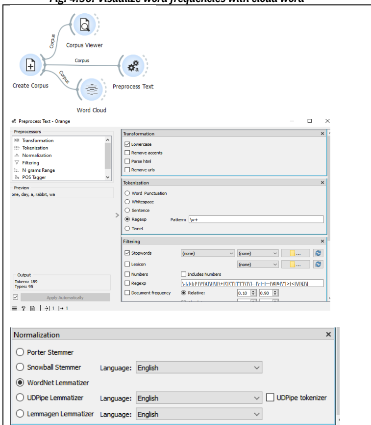
Fig. 4.37: Preprocess Text
