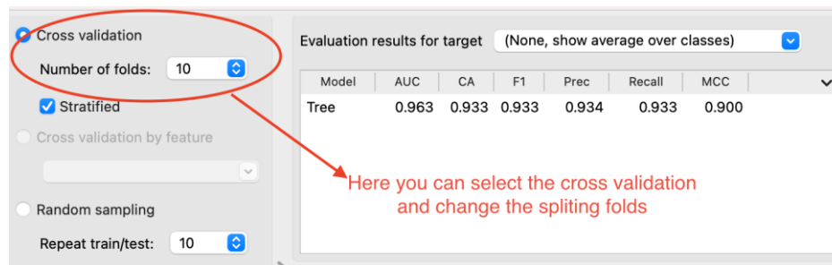
Fig. 4.22
