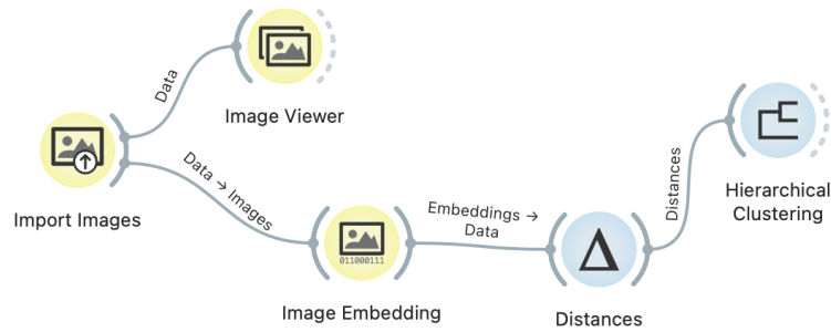
Fig. 4.30: Hierarchical Clustering
